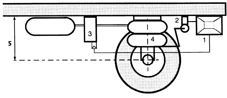
Rys. 10.1. Idea układu ECAS II: 1 – elektronika sterująca; 2 – czujnik wysokości; 3 – zawór magnetyczny; 4 – miech pneumatyczny; 5 – żądana wysokość
